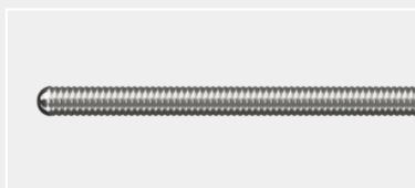
40 cm ナイチノール製ワイヤ (先端部：プラチナタングステン合金コイル)
